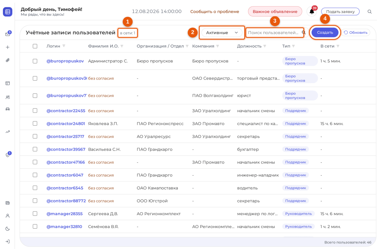
Рисунок 5.1 — Список учётных записей
